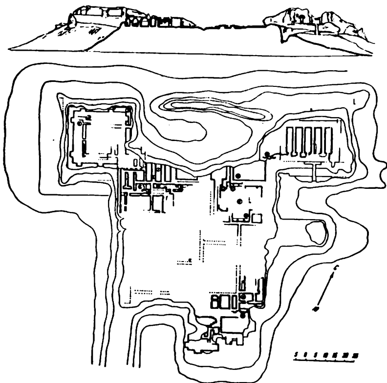
44. ábra. A toprak-kalai palota alaprajza és metszete (détálok).
