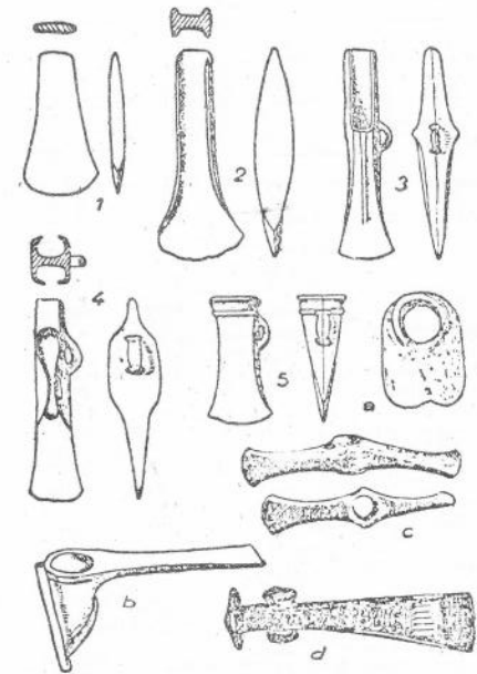
FIG. 1. — Evolución del hacha en la Edad del Bronce. 1 a 5, tipos europeos clásicos: 1, hacha plana; 2, hacha con rebordes; 3, hacha de talón; 4, hacha con alas; 5, hacha de cubo, a a d, tipos de mango vertical: a, azada (Susa); b, azada (Ur); c, hachita-azuela (Hungria); d, hacha de combate (Hungria).
